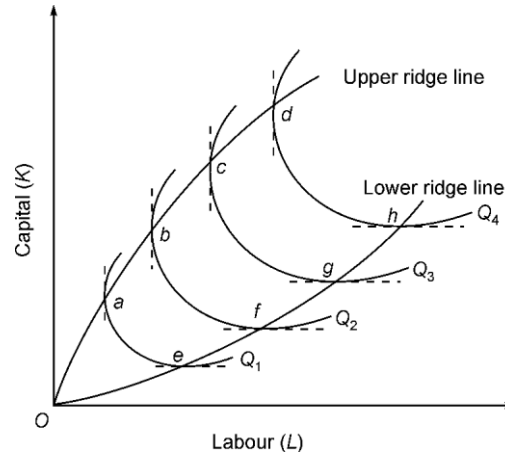
Fig. 2.6 Isoquant Map
