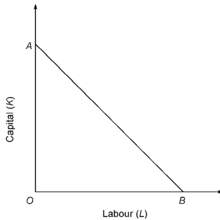
Fig. 2.7 Linear Isoquant
